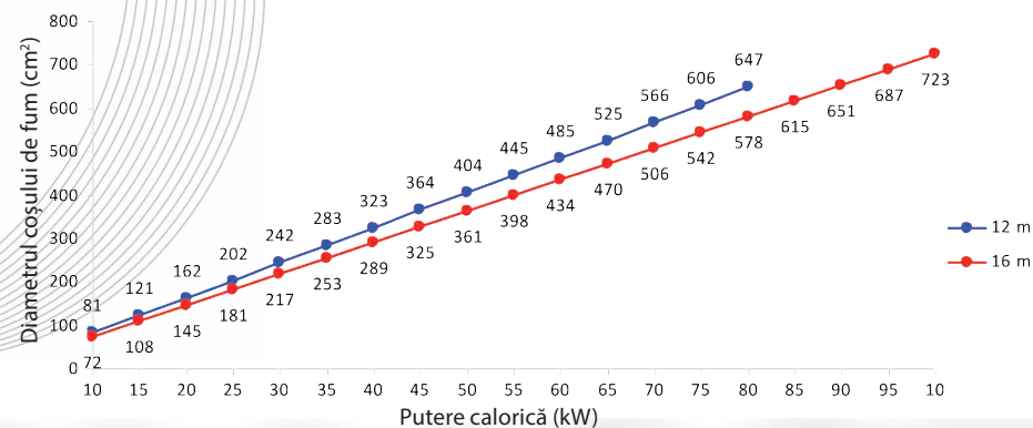
Diagrama nr. 2 Diametrul necesar al coșului de fum în cazul coșurilor de fum de 12, respectiv 16 metri, în funcție de puterea calorică a cazanului
