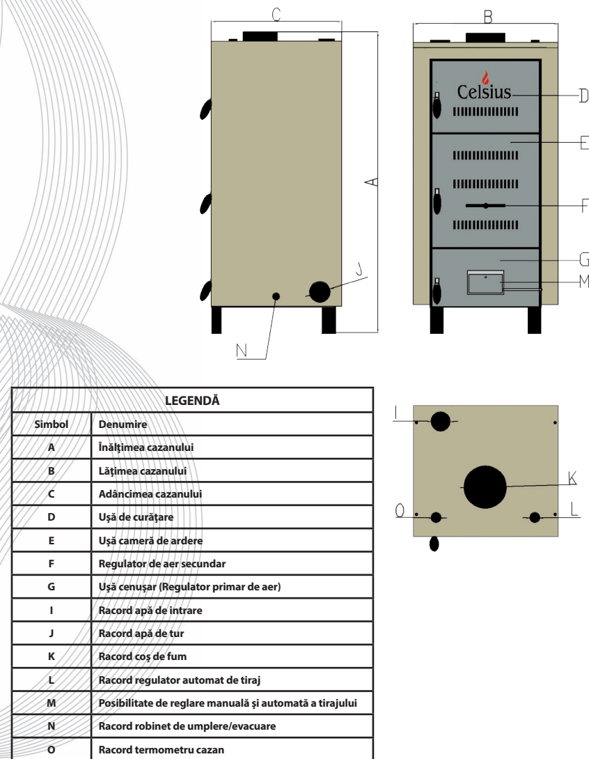
Figura nr. 5 Desenul tehnic al cazanelor Celsius pe combustibil solid
