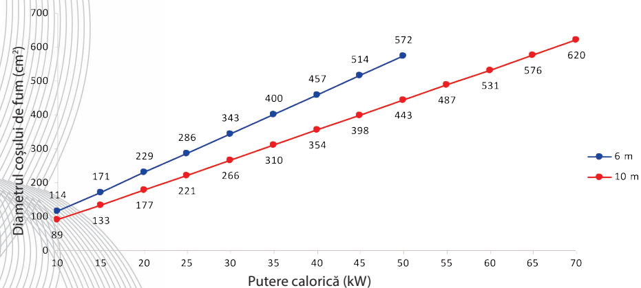
Diagrama nr. 1 Diametrul necesar al coșului de fum în cazul coșurilor de fum de 6, respectiv 10 metri în funcție de puterea calorică a cazanului
